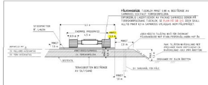
TYPSEKTION ARBETSBÄDD OCH PÅLKRANSUPPSTÄLLNING 150 1410
